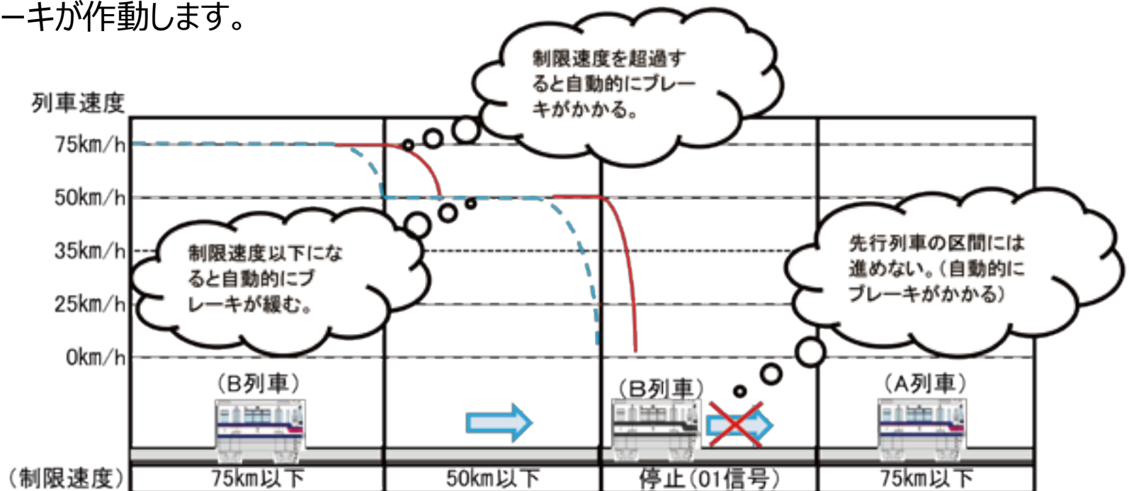
ATC / TD装置説明図
